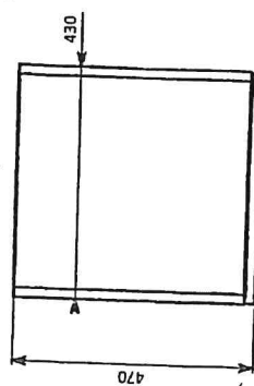
Vista in pianta
